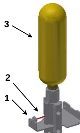
Rys. 14 Jednorazowe narzędzie do uzbrajania.
