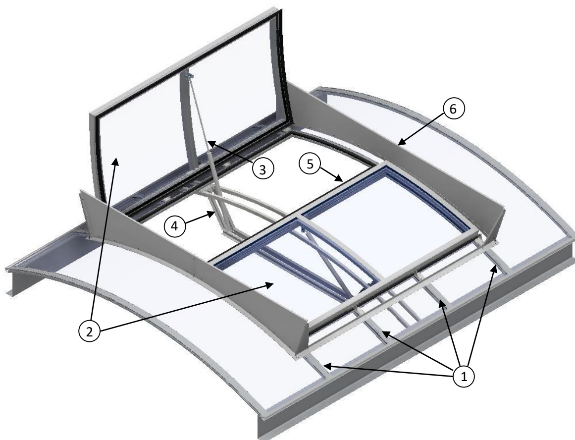
Rys. 1 Budowa klapy oddymiającej mcr PROLIGHT TB zamontowanej w paśmie łukowym mcr PROLIGHT.
