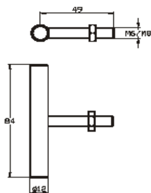
Rys. 6 Śruba 'T'.
