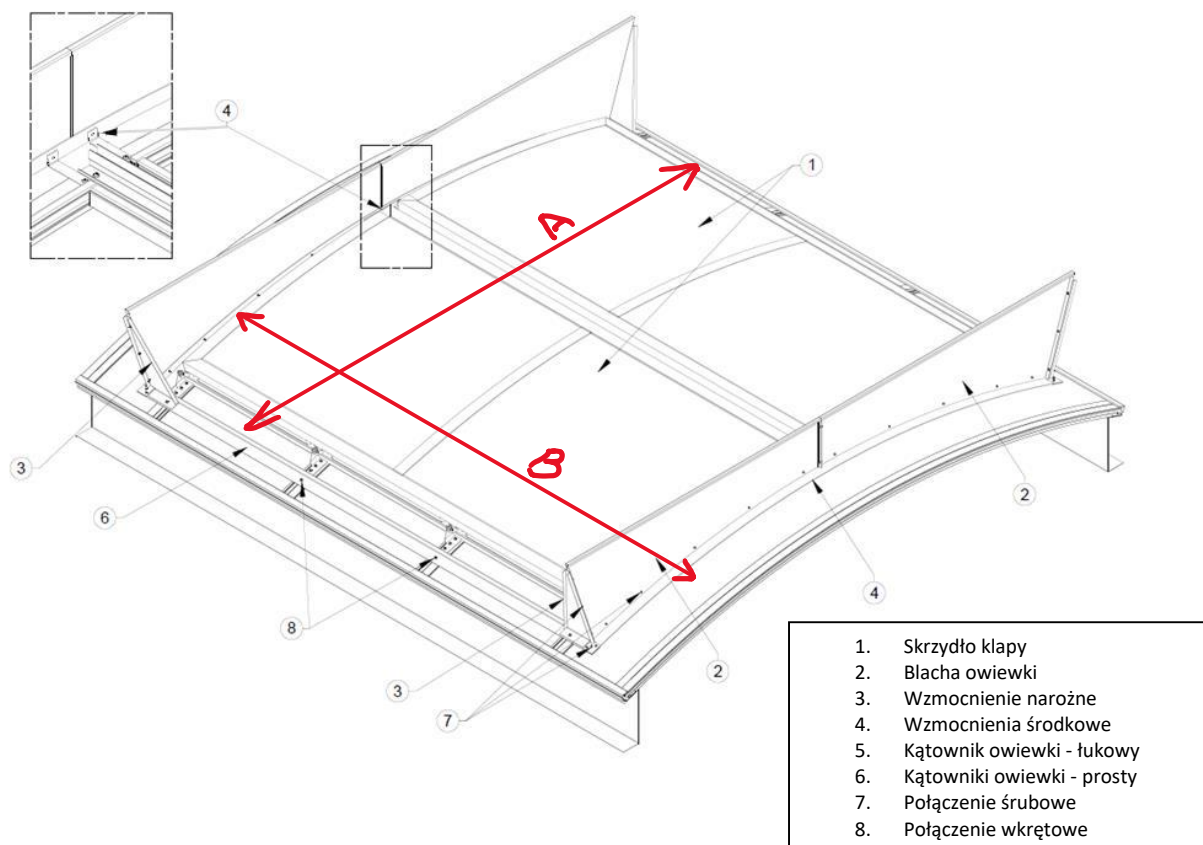
Rys. 5 Owiewki klapy 2-skrzydłowej montowanej na paśmie świetlnym. A – szerokość klapy, B – długość klapy.
